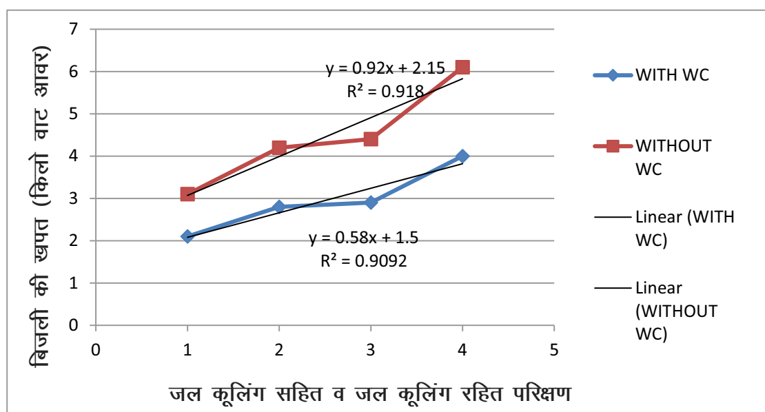
चित्र 3: जल कूलिंग सहित व जल कूलिंग रहित परीक्षणों में बिजली की खपत (किलो वाट आवर)
